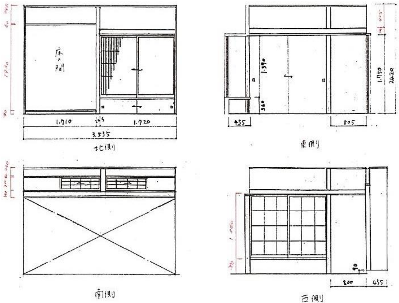
ミニギャラリー平面図・展開図
