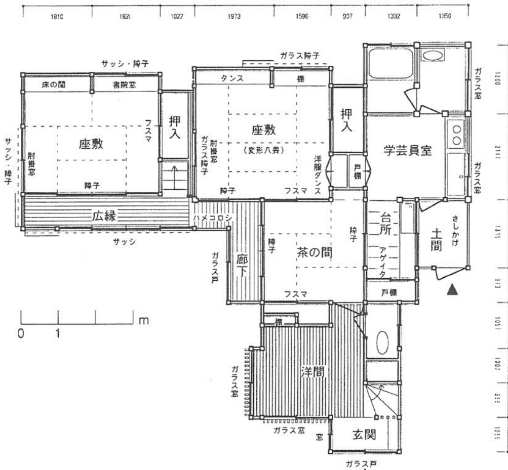
現状1階平面図
