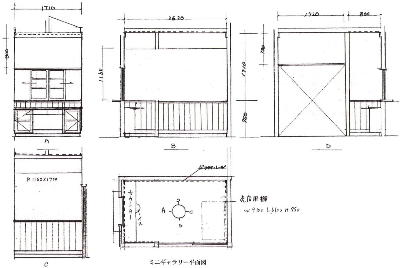
ミニギャラリー平面図・展開図
