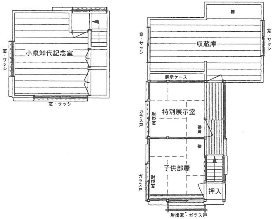
現状2階平面図
